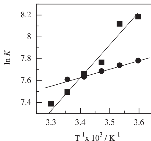
Fig. 5. Temperature dependency of K values of 6-AzaFl· 2 (●) and 6-AzaFl· 3 (■).
